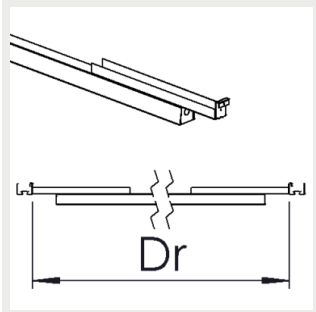
Rampfästen (2)
